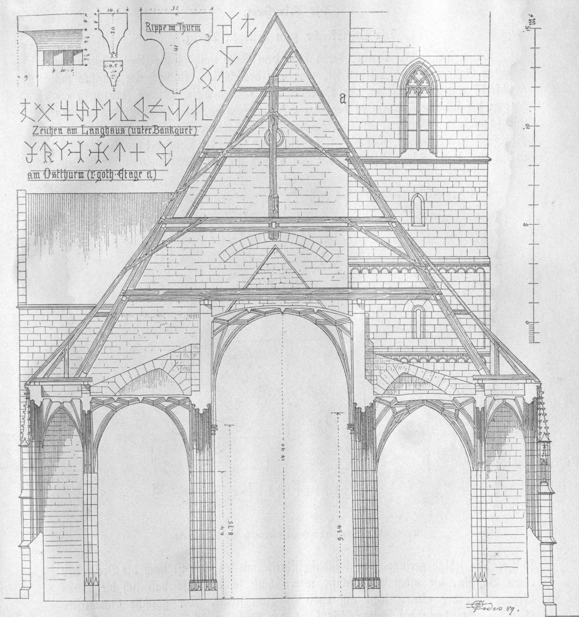
Querschnitt durch die Stiftskirche, mit Blick gegen den alten Ostgiebel.
