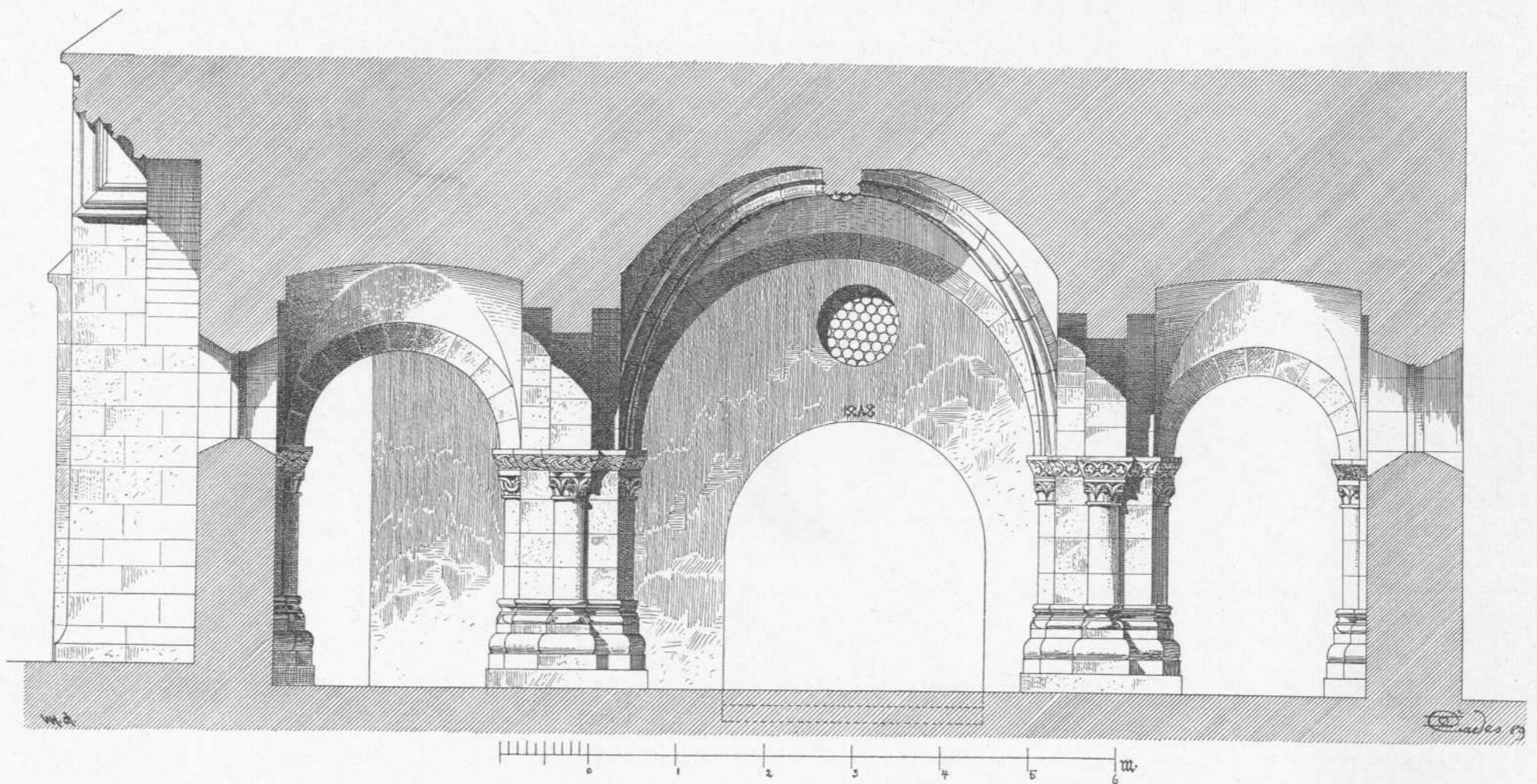
Querschnitt der Vorhalle.
