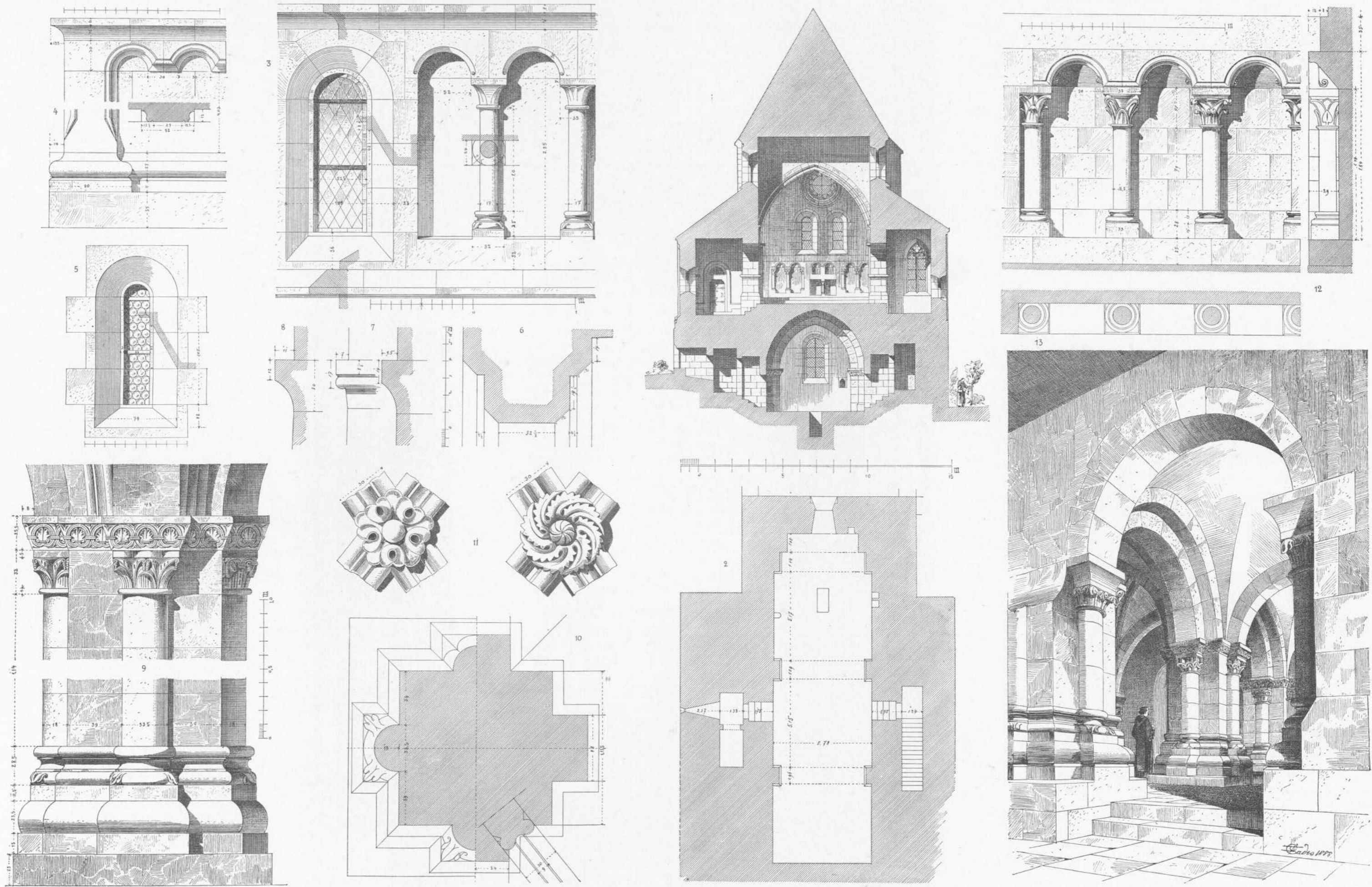
1. Querschnitt durch den Chor. — 2. Grundriss der Krypta. — 3. Arkaden am Mittelschiff (ausen). — 4. Sockel und Dachgesims am nördlichen Seitenschiff. — 5. Fenster am nördlichen Seitenschiff. — 6. Chorbogenprofil. — 7. und 8. Kämpferprofil der Schiffpfeiler. — 9. Vorhallepfeiler. — 10. Grundriss der Vorhallepfeiler. — 11. Gewölbeschlusssteine der Vorhalle. — 12. Wandarkatur. — 13. Blick in die Vorhalle vom nördlichen Seitenschiff aus.
