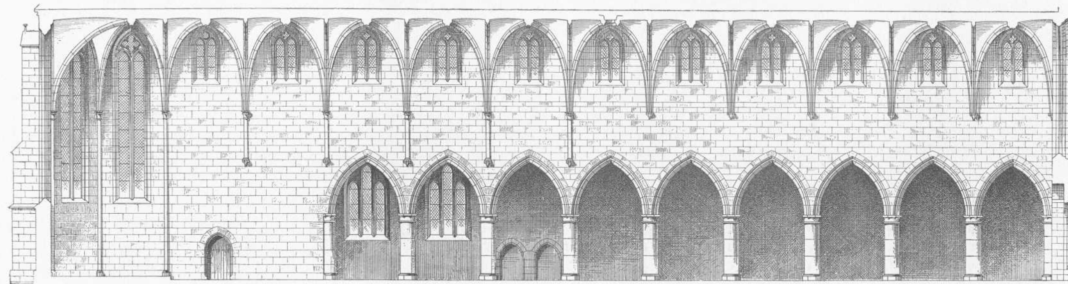
Längenschnitt und Südfassade.
