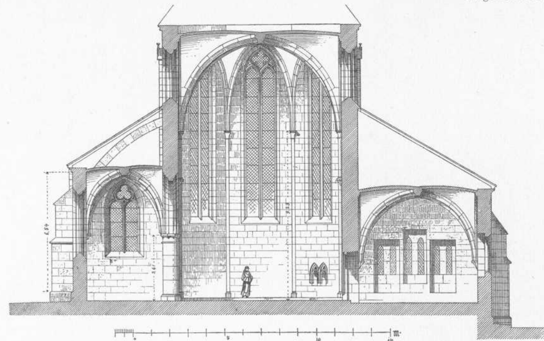
Querschnitt des Chores.
