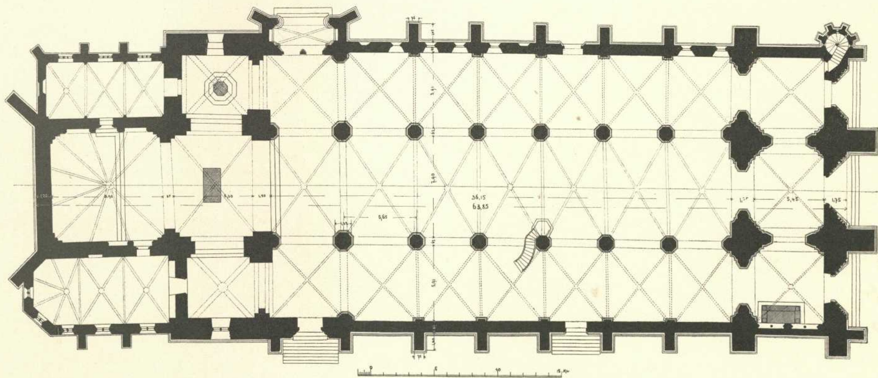
Marienkirche zu Reutlingen. Nordseite, Chor- und Schiff-Querschnitt, Grundriss.
