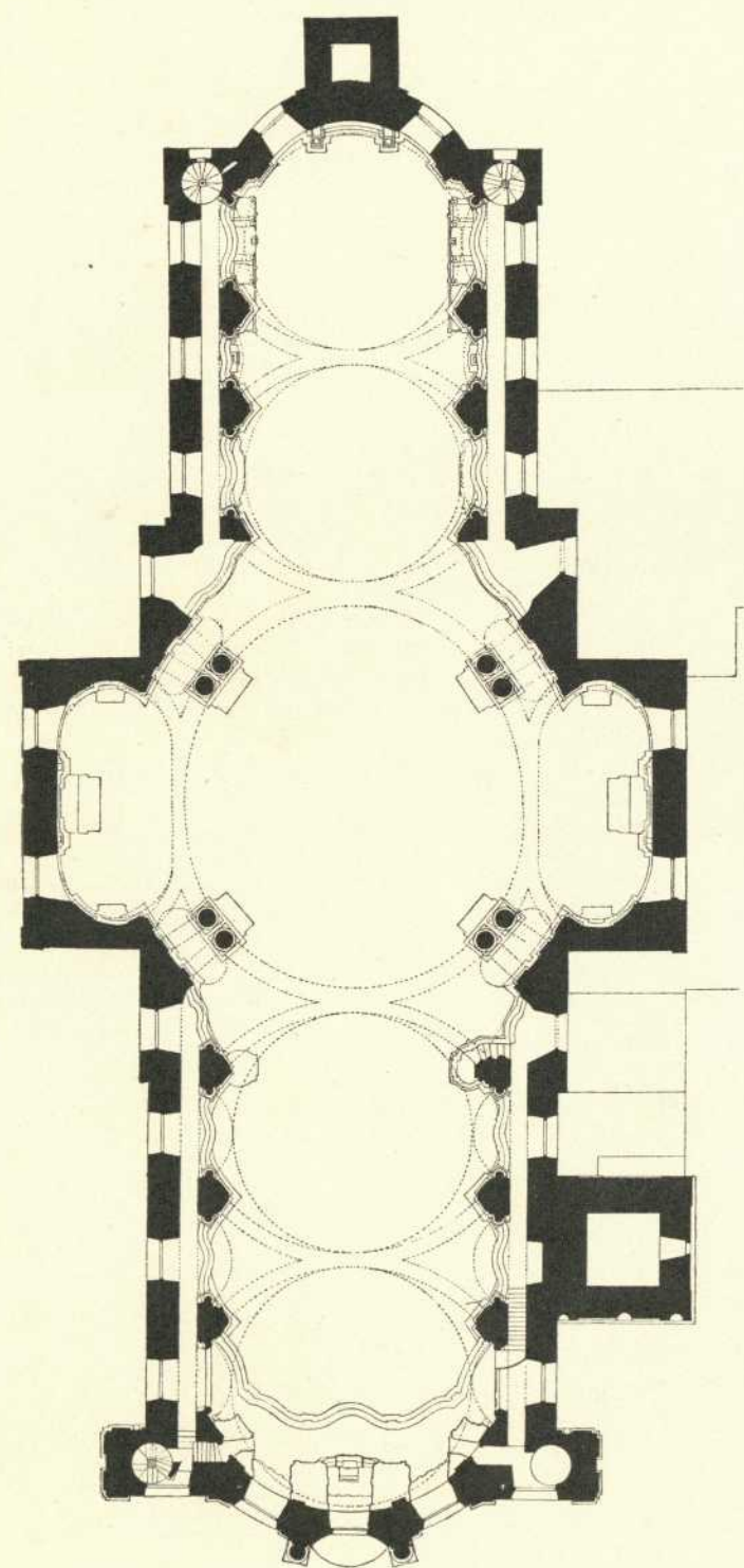
Oberer Grundriss.
