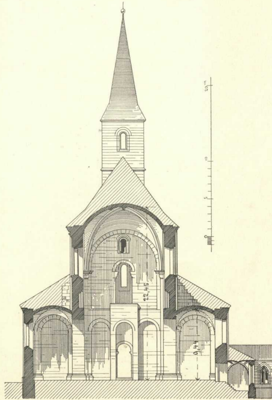
Querschnitt.
