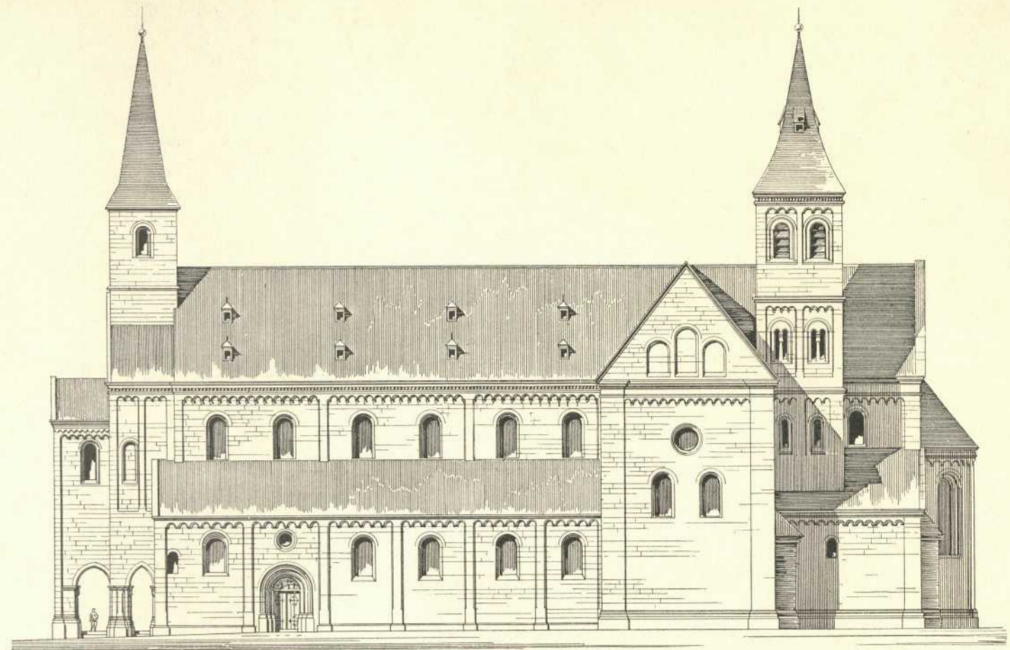
Aufriss von Süden.
