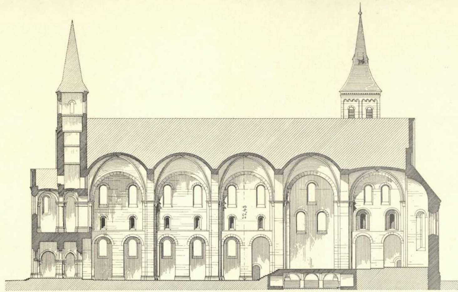
Längenschnitt.
