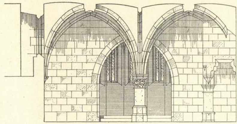
Stiftskapelle. Querschnitt mit Blick in den Chor.
