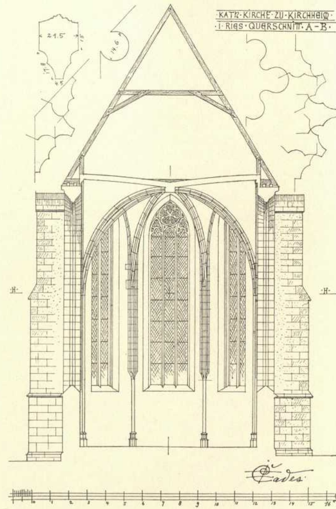
Klosterkirche. Querschnitt und Profile vom Chor.
