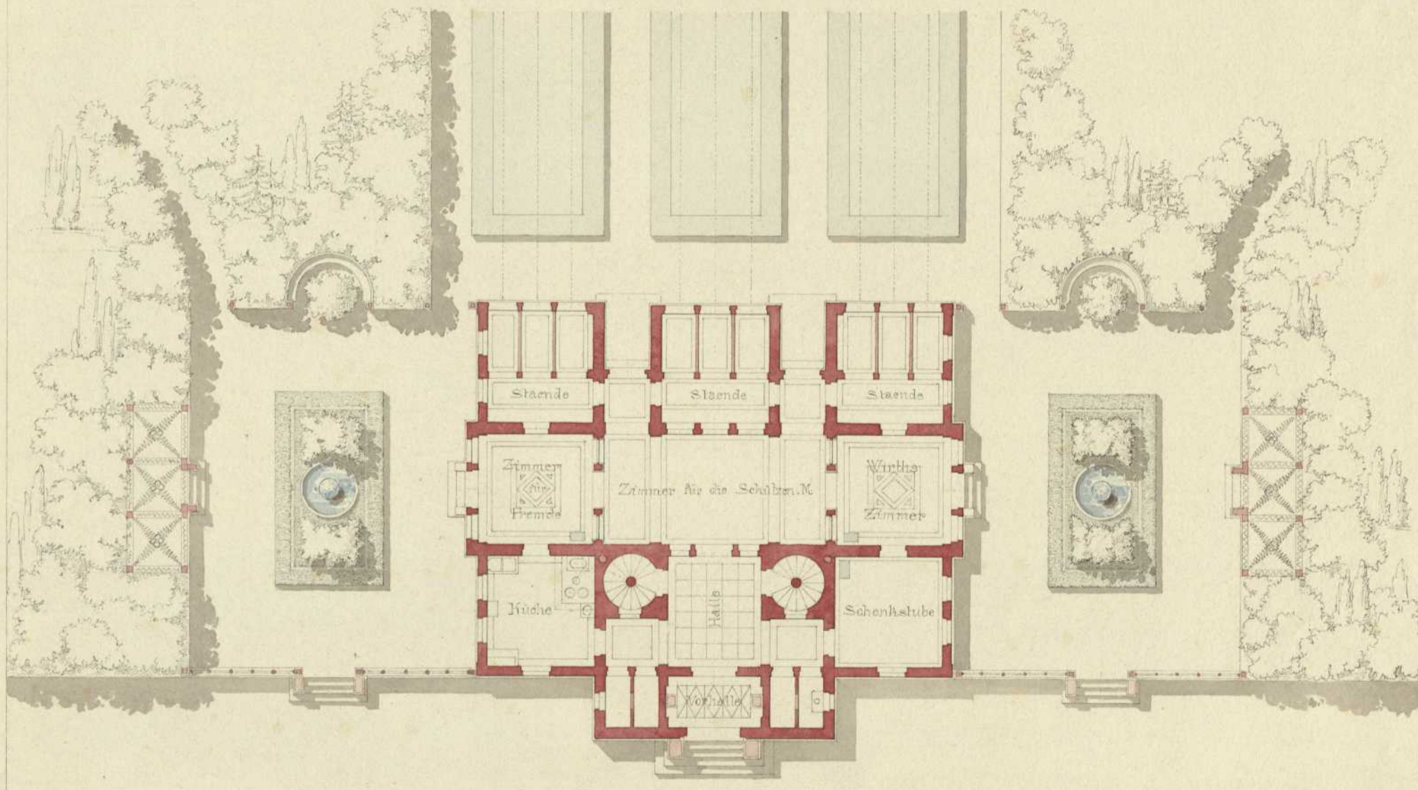
Grundriss des Erdgeschosses
