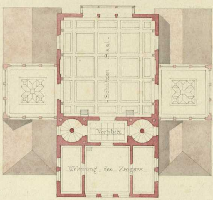
Grundriss des obem Stockes
