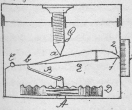
fig II Gehäusekopf
