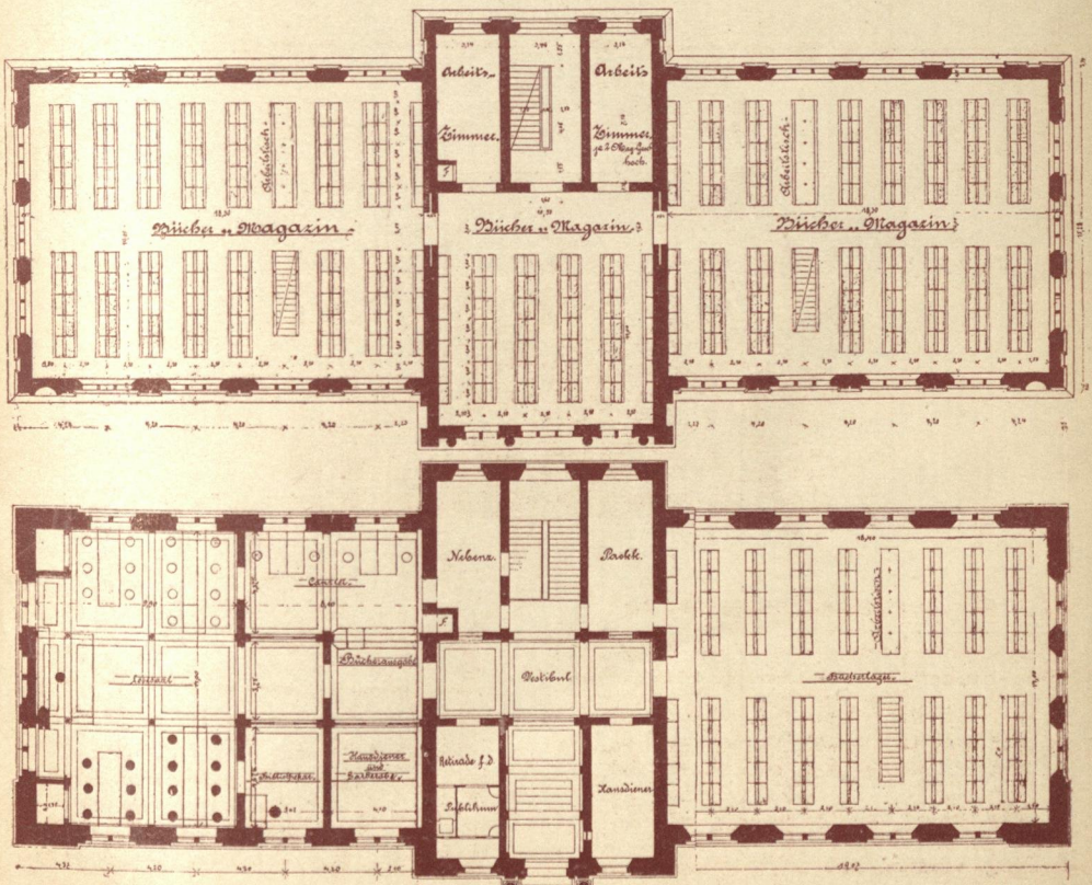
No. 2. Vorentwurf der Hochbau-Inspektion Bremen.
