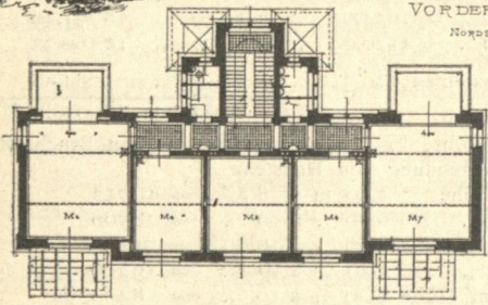
1. Obergeschoss.
