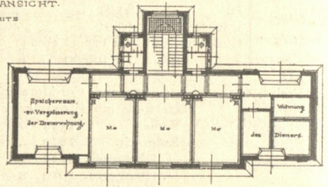
Dachgeschoss.
