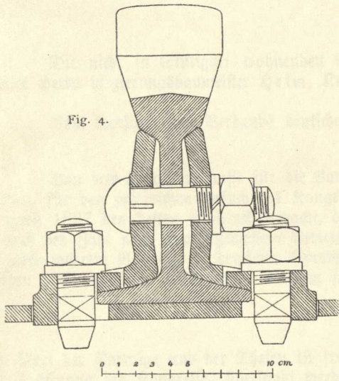
Fig. 4 und 5. Zahnstange.
